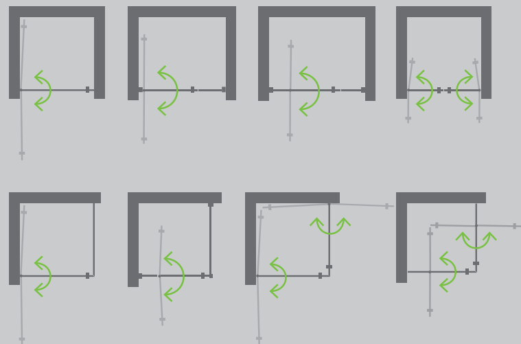
▲ TYP 5617 Drehtür mit Festteil + Badewannenseitenwand
