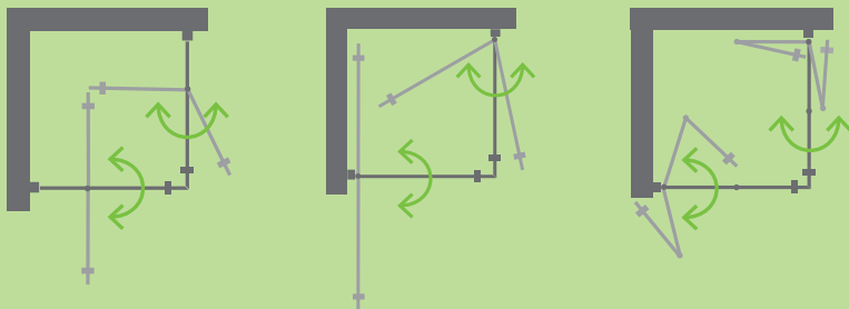
▲TYP 5253 Eckeinstieg Kombination Drehtür mit Festteil + Drehfalttür
